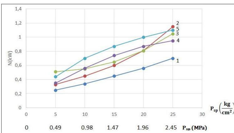
Figura 6. Dependența consumului puterii la frecare de sarcina specifică a lagărului de alunecare axial cu stratul 80% CF-T(II) + 20 TiC în cuplu cu: 1-Grafitofteroplast 7B-2A; 2-APB-200-Б83; 3-CF-T; 4-Grafitofteroplast KB; 5-Fibra de carbon „CYTBAM”.
