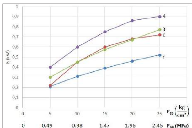
Figura 4. Dependența consumului puterii la frecare de sarcina specifică lagărului de alunecare axial cu stratul CF-T(II) în cuplu cu: 1-Fibra de carbon „CYTBAM”; 2-Grafitofteroplast KB; 3-Cauciuc 7-3825; 4-AMC-3.
