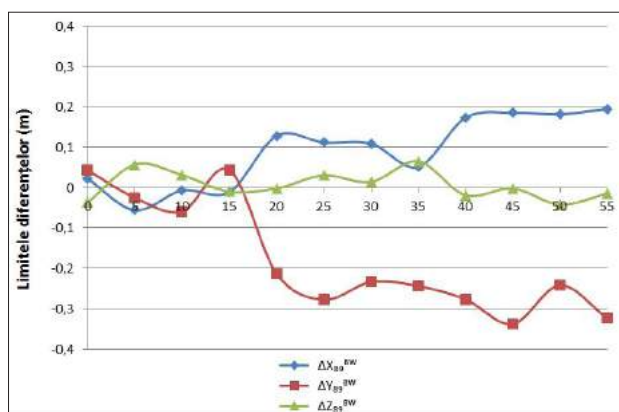
Figura 2. Diferențele \Delta X , \Delta Y , \Delta Z ale punctelor de verificare pentru modelul Bursa – Wolf.
