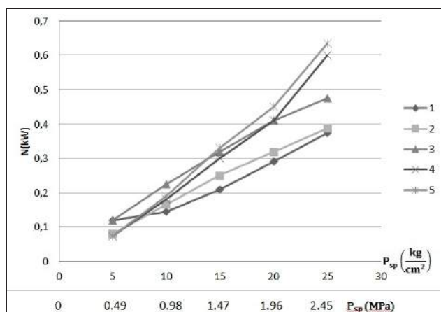
Figura 1. Dependența consumului puterii la frecare de sarcina specifică a lagărului de alunecare axial cu stratul ПН55Т45 în cuplu cu: 1-Grafită APB-200-B83; 2-CF-T; 3-Cauciuc 7-3825; 4-Grafitofteroplast KB; 5-Grafitofteroplast 7B-2A;
