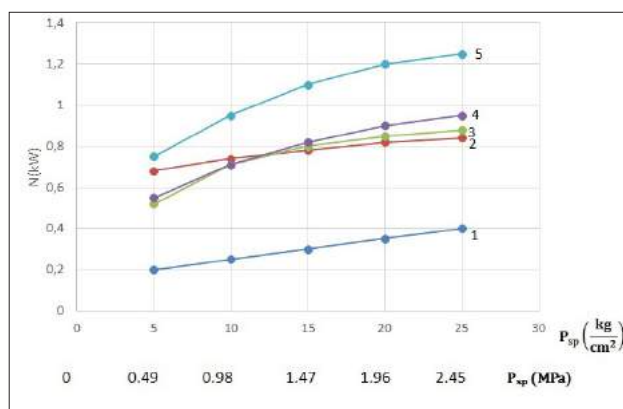
Figura 3. Dependența consumului puterii la frecare de sarcina specifică a lagărului de alunecare axial cu stratul 50% ПН55Т45+TiC în cuplu de frecare cu: 1-CF-T; 2-Grafitofteroplast KB; 3-АГ-1500-Б83; 4-APB-200-Б83; 5-Grafitofteroplast 7B-2A.
