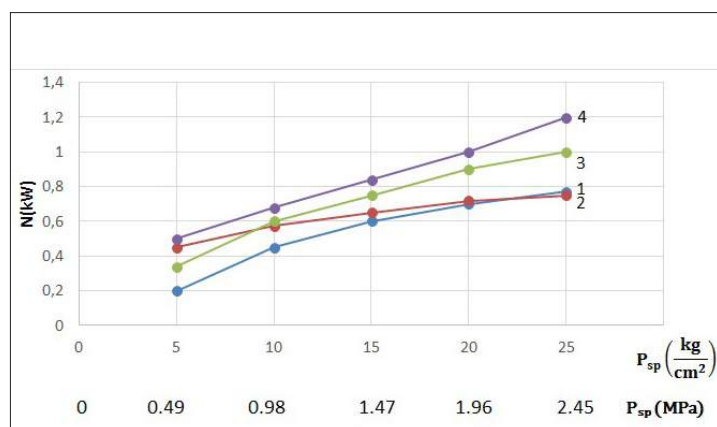
Figura 5. Dependența consumului puterii la frecare de sarcina specifică a lagărului de alunecare axial acoperit cu pulbere CF-T(II) în cuplu cu: 1-APB-200-Б83; 2-CF-T; 3- Grafitofteroplast 7B-2A; 4-АГ-1500-Б83;
