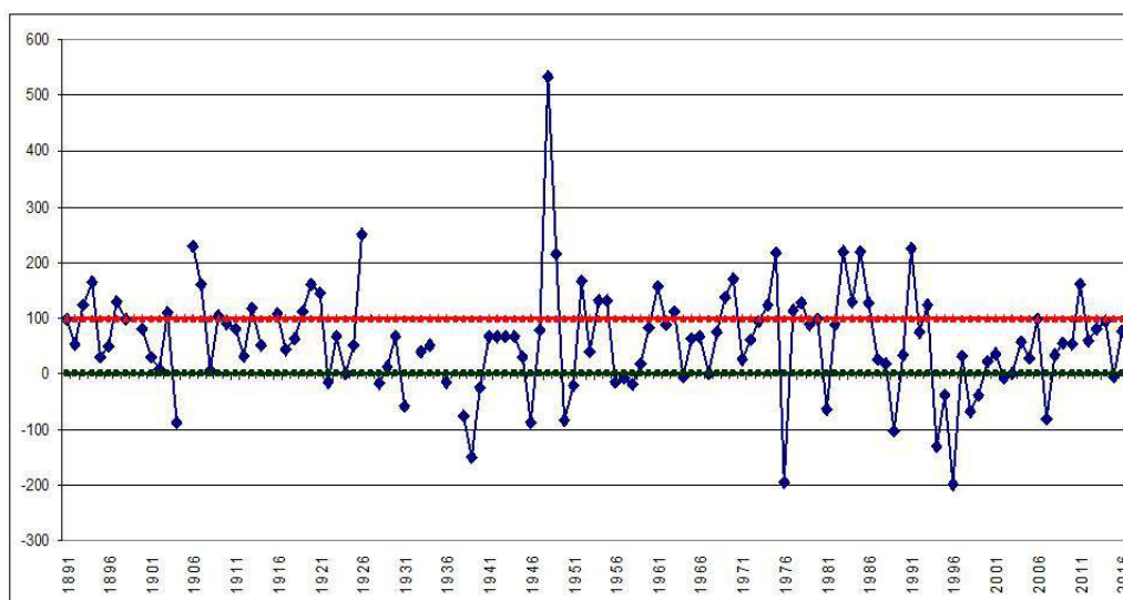
Figura 2. Mersul multianual al Indicelui Diekman, st. Chișinău (1891–2016)
