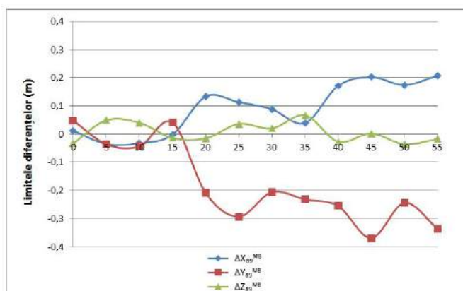
Figura 3. Diferențele \Delta X , \Delta Y , \Delta Z ale punctelor de verificare pentru modelul Molodensky – Badekas.
