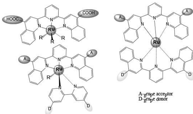
Figura 1. Structura compușilor coordinativi ai ruteniului tridentati și mixdentati.
