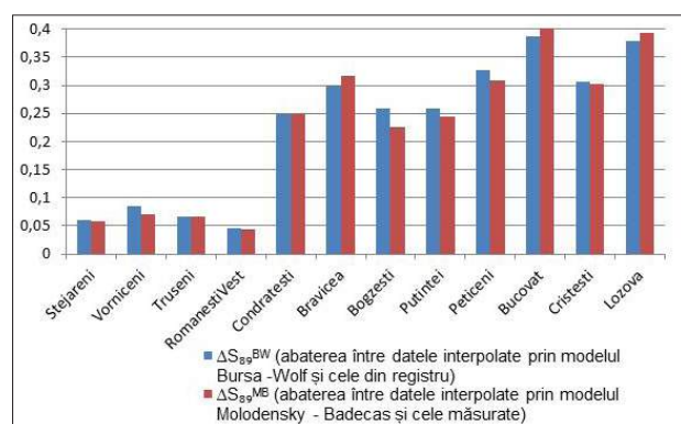
Figura 4. Abaterile \Delta S drept rezultat al utilizării gridului de interpolare.
